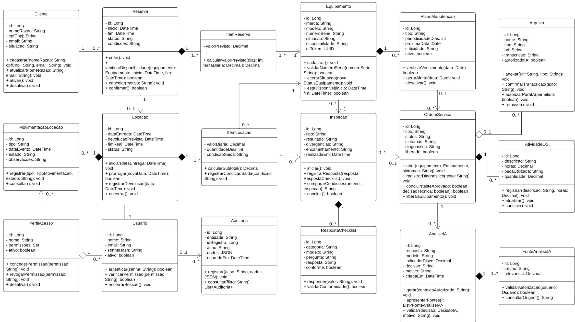
DIAGRAMA DE CLASSES
